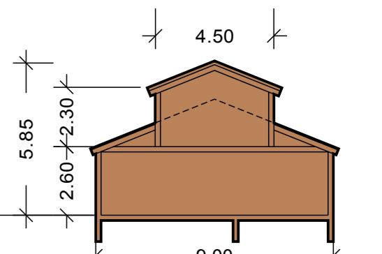
KENNISNIÐ MKV 1:200 BYGGINGARREITUR D
