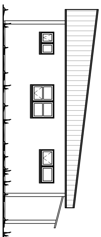
ÚTLIT AUSTUR 1:100
