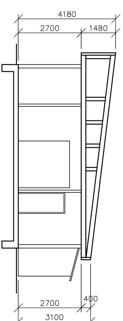
SNID A-A 1:100
